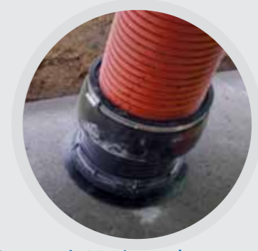
Piquage à 90° (manchon souple) DN 100, 160, 200 & 250mm Collecteur à paroi épaisse 21 - 150mm DN 250 - 1500mm
